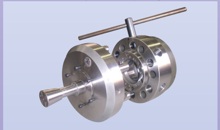
Modulares System für ID/AD-Spannzangen
